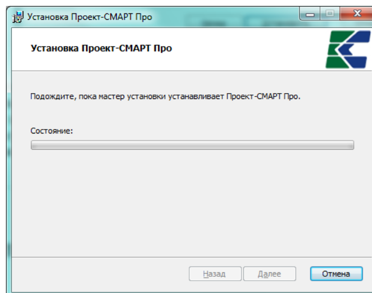
Рисунок 7. Процесс установки
