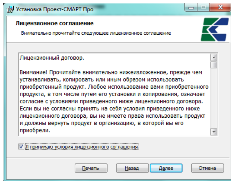
Рисунок 3. Лицензионное соглашение
