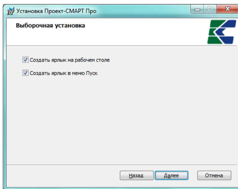
Рисунок 5. Выборочная установка
