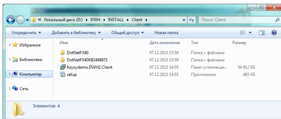
Рисунок 1. Структура каталога
